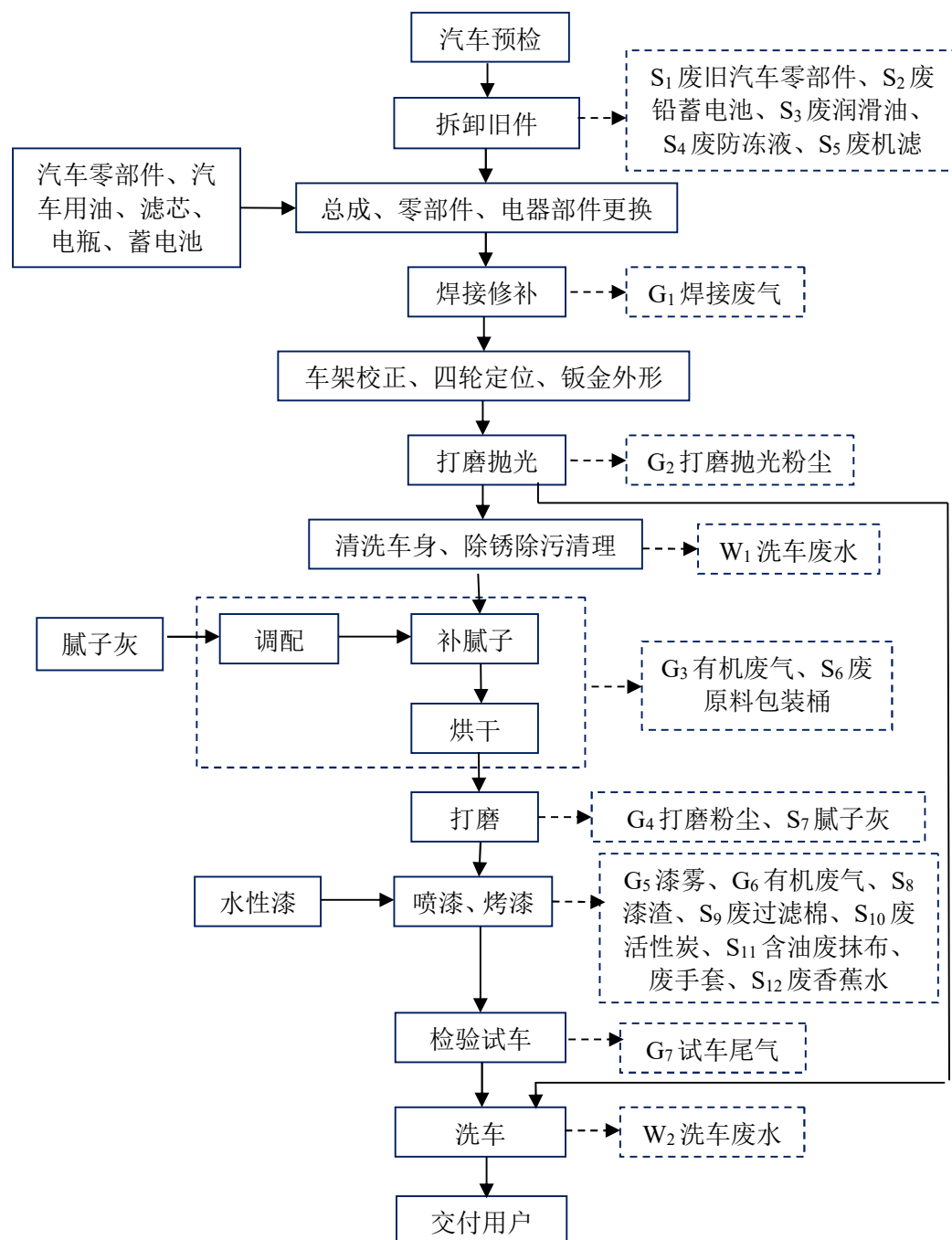
图 3.4-1 验收项目工艺流程及产污环节图
